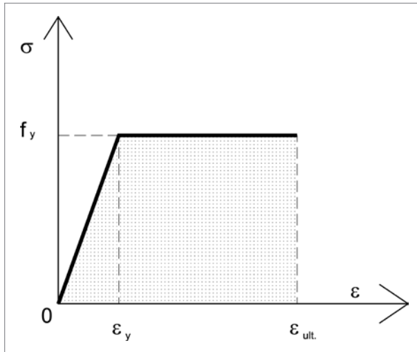
Figura 4.2. Materiale elasto-plastico
