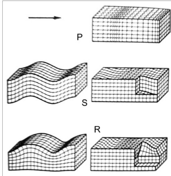
Figura 9.2. P = onde longitudinali; S = onde di taglio; R = onde di Raleigh (Cestelli Guidi 1 )
